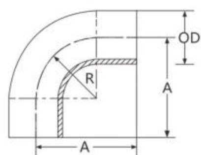
90°卡焊式长弯头 90-deg clamp long elbow
