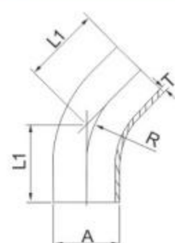
BPE管道 BPE Tube
