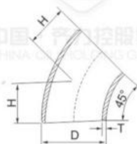
45°弯头 45°Elbow
