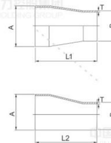
同心大小头 加长型 Long concentric Reducer
