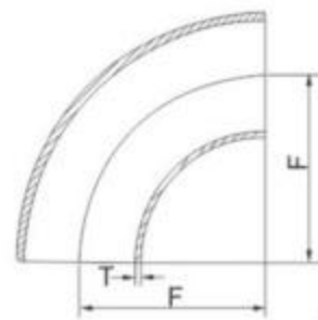
90°弯头 90°Elbow
